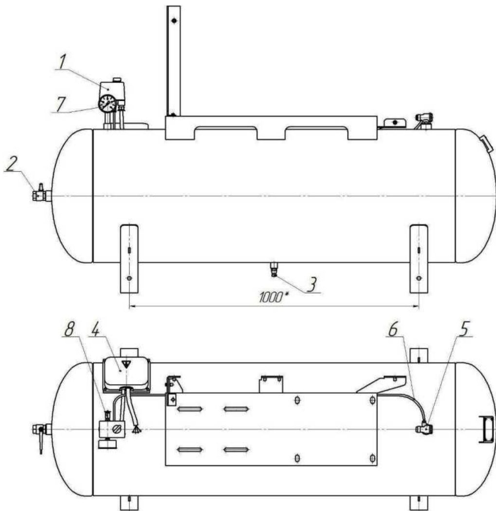
Рис.9 Ресивер, модель С415М, С415М-01, С415М-02
