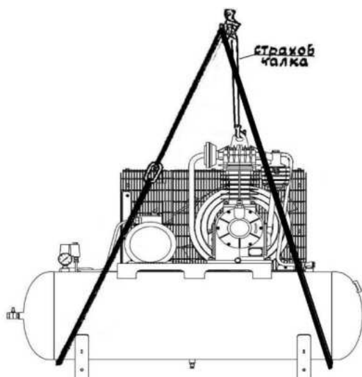
Рис.21 Схема строповки компрессора модель C415M, C415M-01, C415M-02
