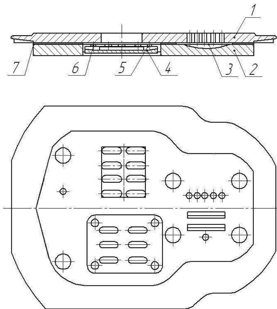
Рис.8 Блок клапанный:
