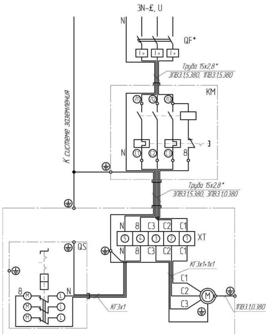
Рис.19 Схема электрическая принципиальная и соединений компрессора, модель C415M-02
