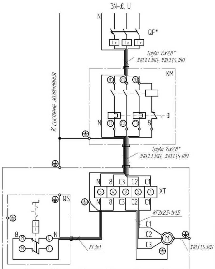
Рис.18 Схема электрическая принципиальная и соединений компрессора, модель C416M, C416M-01
