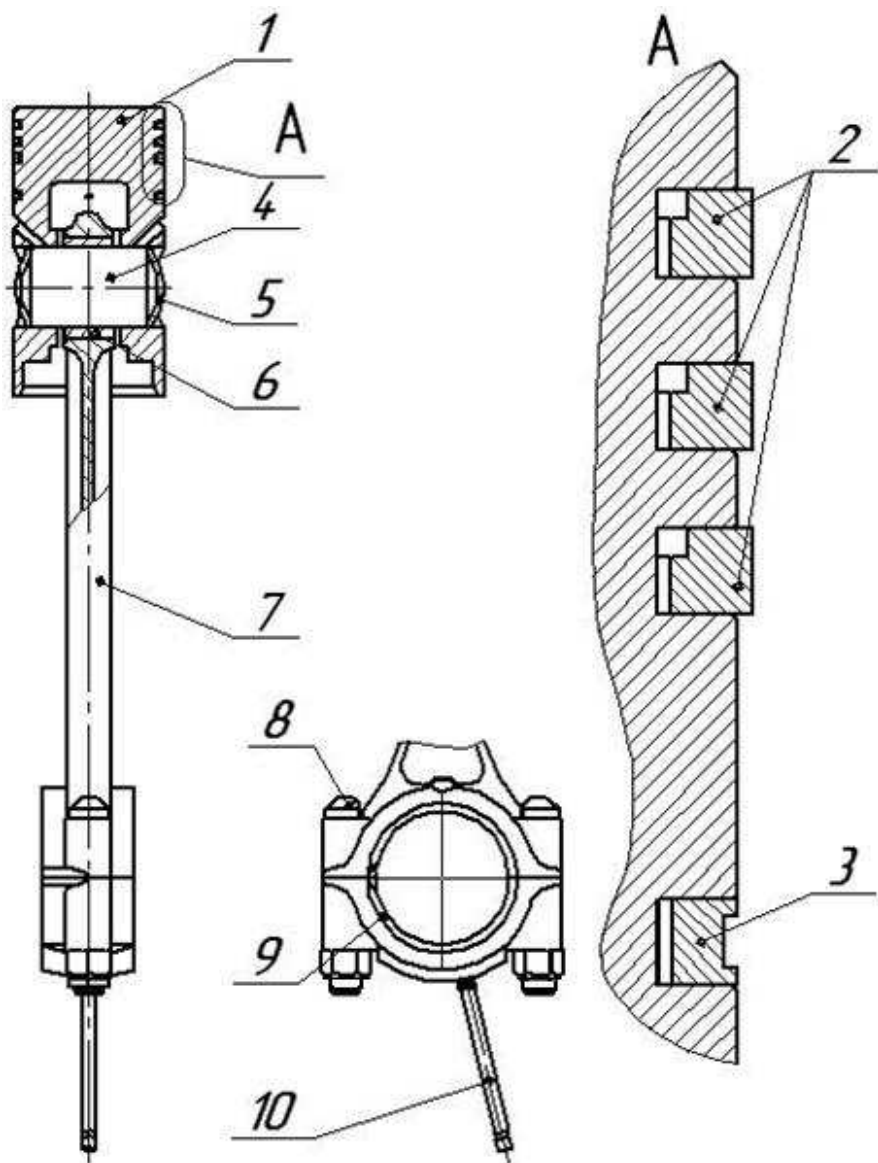
Рис.7 Поршень цилиндра высокого давления:
