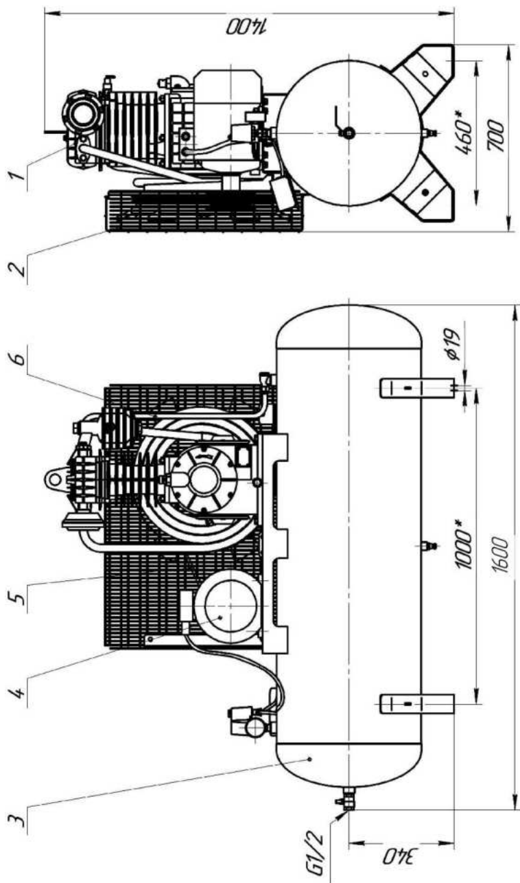
Рис. 1 Компрессор, модель С415М, С415М-01, С415М-02
