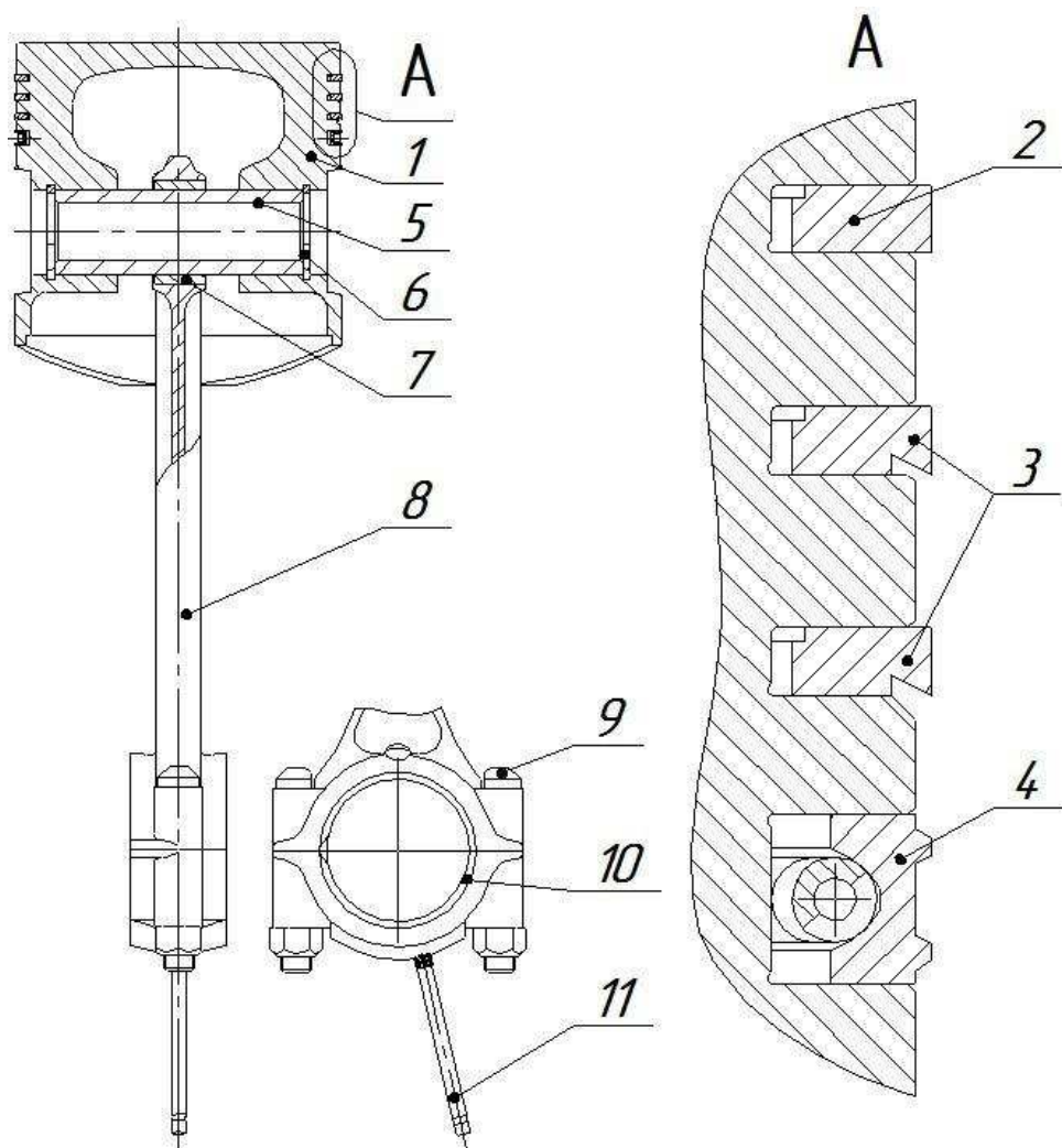
Рис.6 Поршень цилиндра низкого давления:
