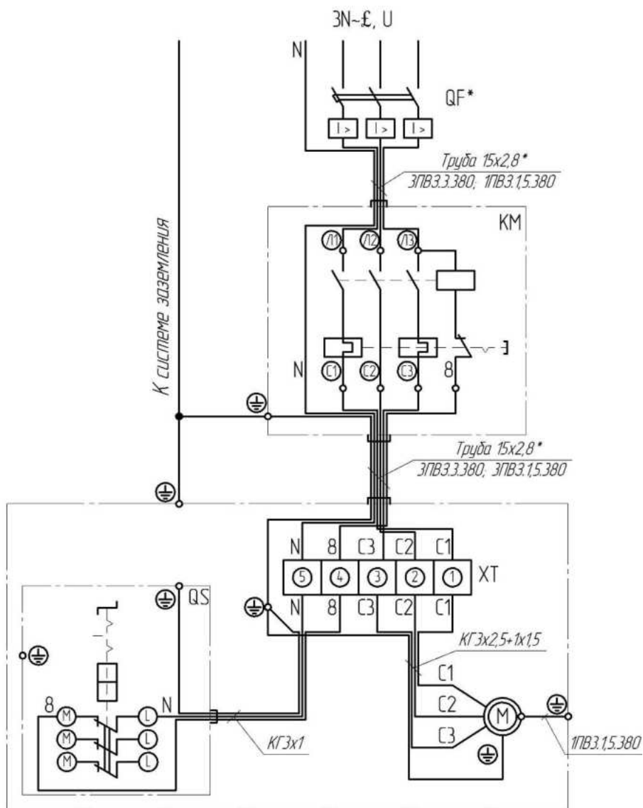
Рис.20 Схема электрическая принципиальная и соединений компрессора, модель C416M-02
