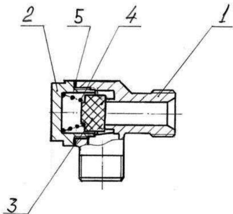
Рис. Рис.11 Клапан обратный
