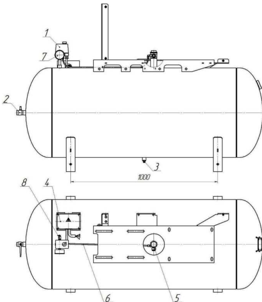
Рис.10 Ресивер, модель С416М, С416М-01, С416М-02
