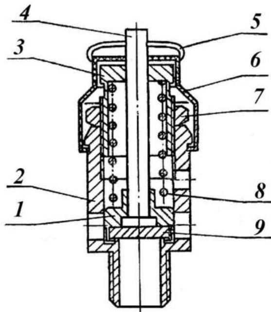
Рис.13 Клапан предохранительный на ресивере
