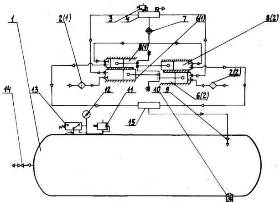
Рис. 16 Схема пневматическая принципиальная компрессора, модель С416М, С416М-01, С416М-02
