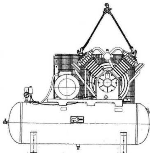
Рис.22 Схема строповки компрессора модель C416M, C416M-01, C416M-02
